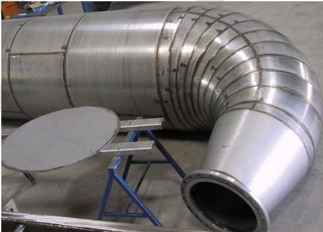
Beschleunigungsbogen DN 900 Werkstoff 1.4571
