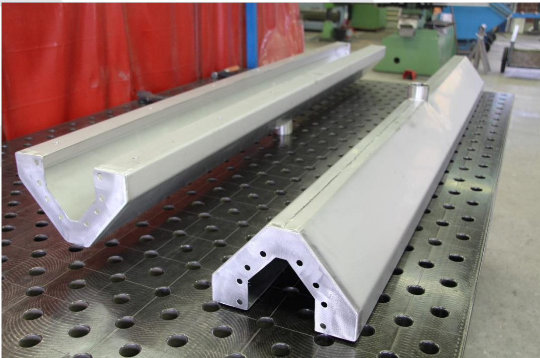
2-teilige Rücklaufwanne für Leim, Werkstoff-Nr. 1.4571
