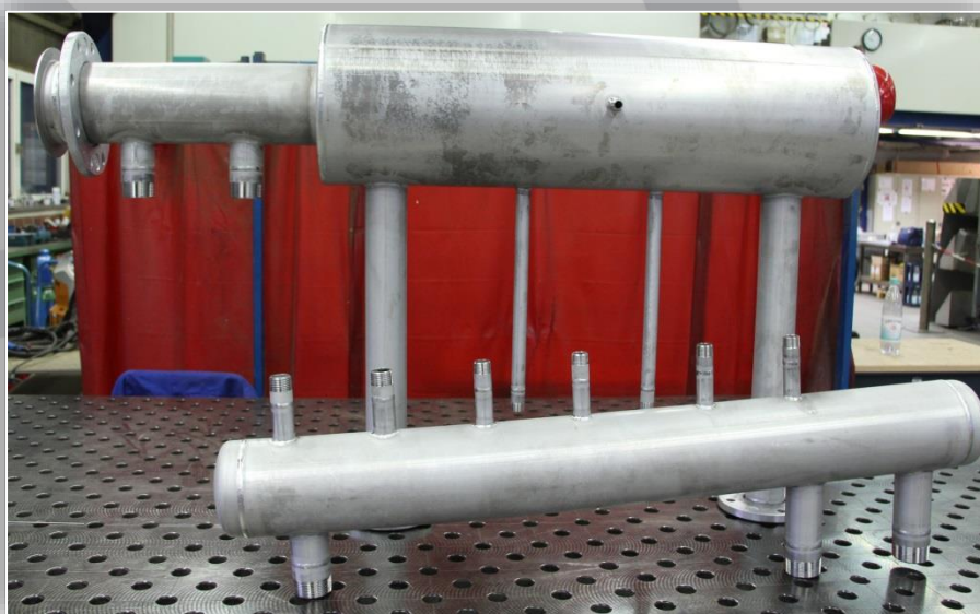
Kühlwasserverteiler für die Stahlindustrie, Werkstoff 1.4571, DN 250 bzw. DN 150
