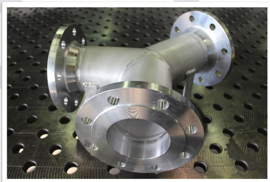
Hosenstück DN 100/ PN 16, Werkstoff: 1.4571
